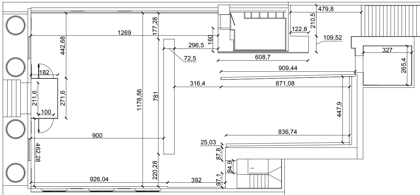
PLANTA COTADA 1:150
